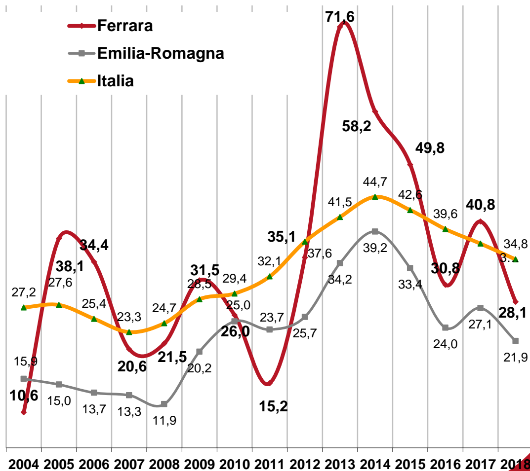
Trend temporale
